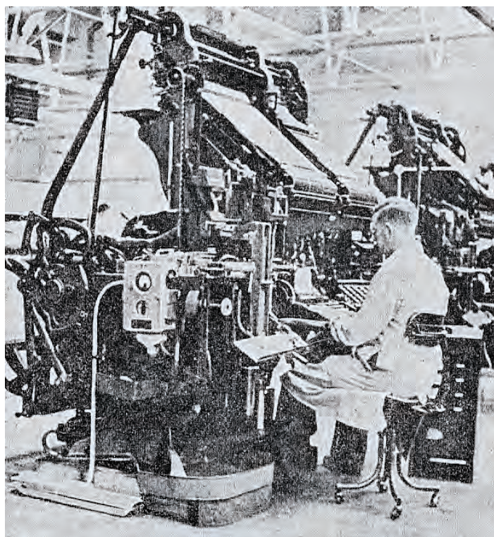
77. Linotyp
