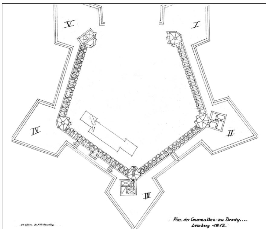
43. Plan der Casamatten zu Brody, Lemberg 1812. Kopia ze zbioru DrA. Czołowskiego. IS PAN nr inw. 7698.
