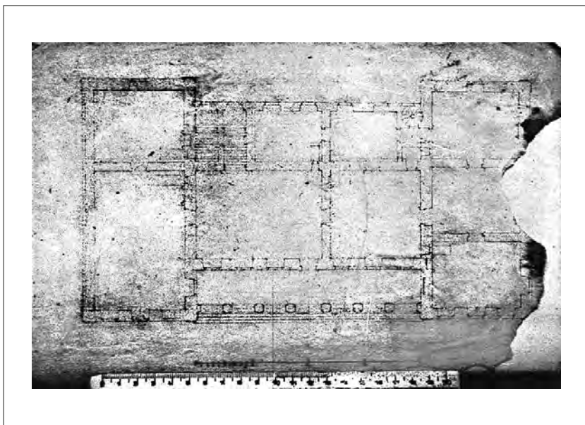
148. Warszawa, plan przyziemia pałacu Koniecpolskich z ok. II poł. XVII w. (wg Krótką nauka budowniczą dworów, pałaców, zamków podług nieba i zwyczaju polskiego , opr. A. Miłobędzki, Wrocław 1957, ryc. 30).
