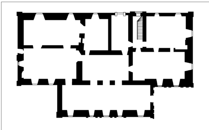
37. Potok, pałac, hipotetyczna rekonstrukcja planu parteru (opr. B. Smoczyński, wg A. Barczyk, Pałac Raczyńskich w Złotym Potoku. Źródła do dziejów architektury i wyposażenia , w: Historia – konserwacja – rewitalizacja. Funkcjonowanie rezydencji regionu łódzkiego w kontekście doświadczeń europejskich. Prace dedykowane pamięci Profesora Leszka Kajzera , Łódź 2016, s. 100, il. 1).
