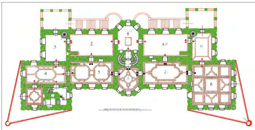
137. Podhorce, pałac, plan pierwszego piętra, rysunek ram stropów (wg A. Szyszko-Bohusz, Podhorce , w: „Sztuki Piękne”, t. 1, 1924–1925, s. 152, opr. B. Smoczyński).
