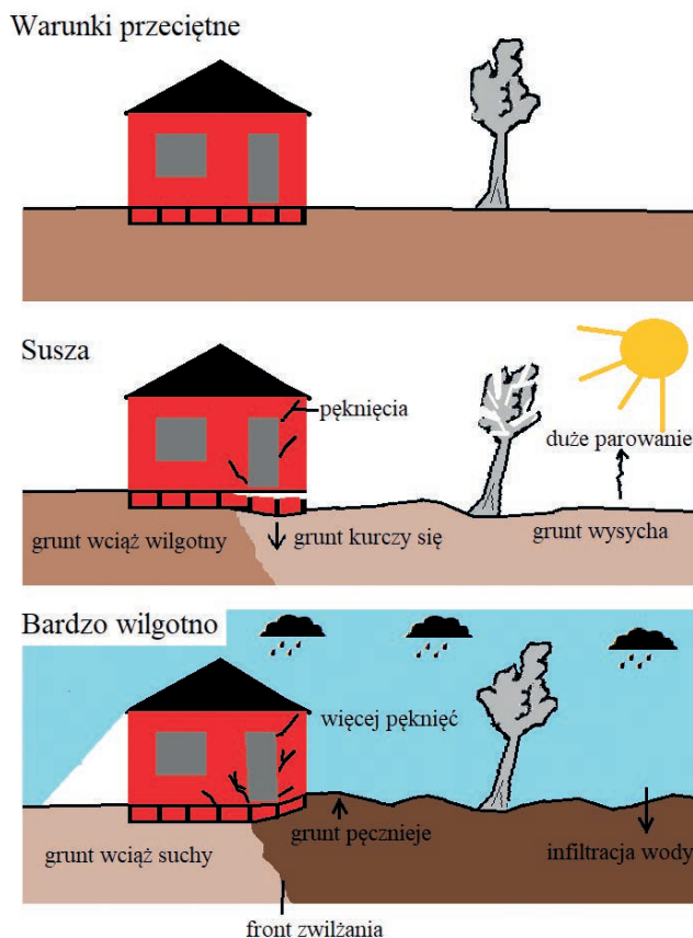
Ryc. 6. Schemat przedstawiający wpływ naprzemiennego wysychania i nawilżania gruntów ilastych na zabudowę
