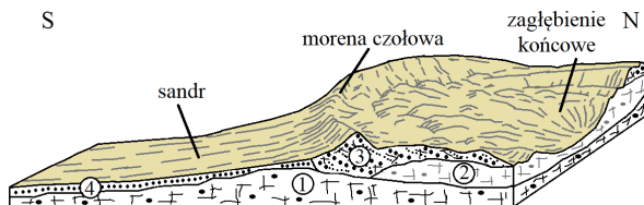
Ryc. 19. Morena czołowa na tle form sąsiadujących i schemat budowy litologicznej 1 – glina zwałowa starsza, 2 – glina zwałowa młodsza, 3 – piaski, żwir i gliny akumulacji czołowomorenowej, 4 – piaski i żwir sandrowe
