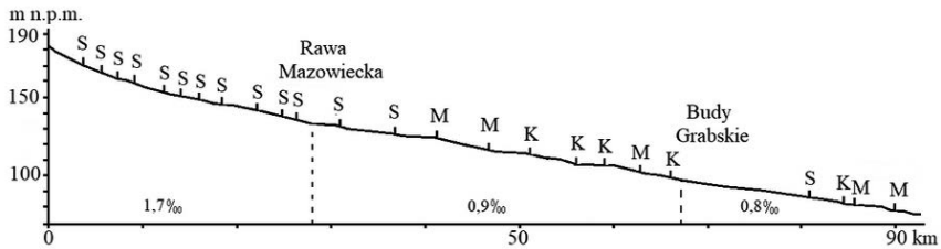
Ryc. 64. Lokalizacja młynów wodnych na Rawce w środkowej Polsce, stan na początku XX w. S – młyn ze stawem młyńskim, M – młyn na młynówce, czyli sztucznie ukształtowanym kanale zasilanym wodą z rzeki, K – młyn na podpiętrzonej korycie, 1,7‰ – spadek rzeki
