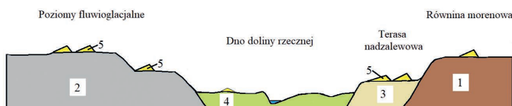
Ryc. 88. Najczęstsze miejsca występowania wydm śródlądowych 1 – glina zwałowa, 2 – piaski i żwiry fluwioglacjalne, 3 – piaski i mułki fluwioperyglacjalne, 4 – piaski i namuły den dolinnych, 5 – piaski eoliczne w wydmach
