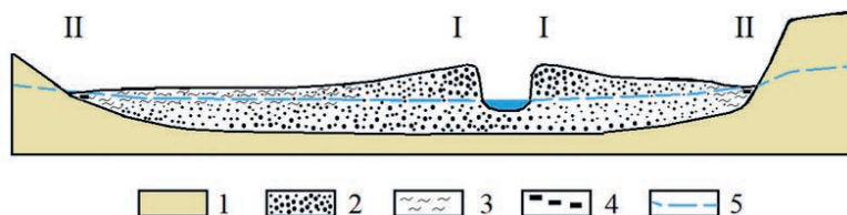
Ryc. 63. Przekrój poprzeczny przez terasę zalewową I – wał przykorytowy, II – strefa przystokowa, często zatorfiona, 1 – osady starsze od utworów terasy zalewowej holocenińskiej, 2 – piaski różnoziarniste, 3 – namuły aluwialne, 4 – torfy, 5 – poziom wód aluwialnych
