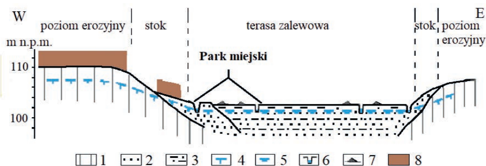
Ryc. 80. Położenie Łęczycy w obrębie doliny Bzury. Zamek i zabudowa miejska na poziomie erozyjnym zbudowanym z gliny, a park miejski na terasie zalewowej 1 – glina morenowa, 2 – piaski terasy nadzalewowej i stokowe, 3 – piaski i mulki terasy zalewowej, 4 – poziom wód gruntowych, śródglinowych, 5 – wody aluwialne, 6 – rzeka i rowy odwadniające, 7 – wały przeciwpowodziowe, 8 – zabudowa miejska
