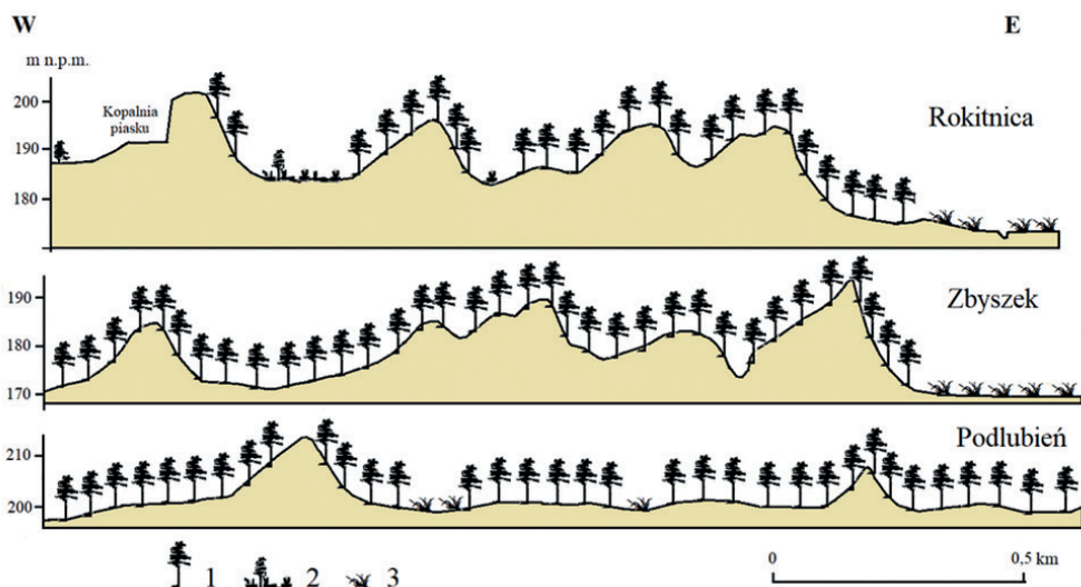
Ryc. 100. Urozmaicona rzeźba na obszarach wydmych w południowej części województwa łódzkiego 1 – lasy sosnowe, 2 – roślinność torfowisk, 3 – trawy
