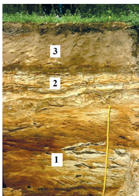
Ryc. 61. Budowa terasy zalewowej na przykładzie doliny Rawki 1 – osady piaszczysto-żwirowe akumulowane w korycie rzecznym (osady korytowe), 2 – piaszczysto-mułkowe osady akumulowane na odsypie meandrowym i osady powodziowe, 3 – osady piaszczysto-mułkowe powodziowe przekształcone przez procesy glebowe
