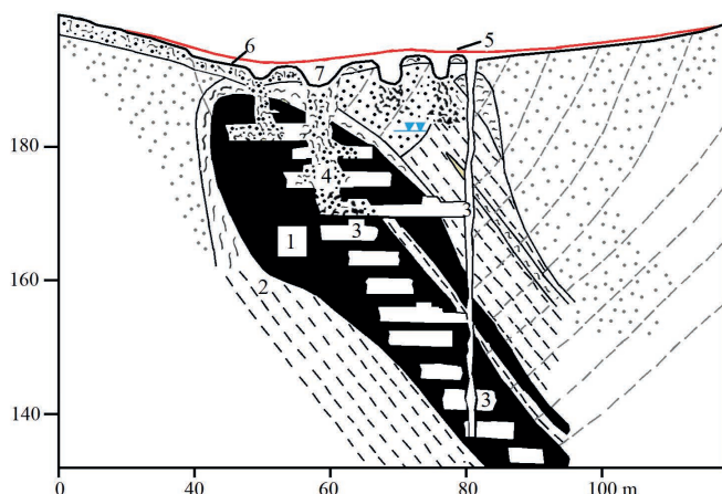
Ryc. 25. Szkic budowy geologicznej fragmentu moreny czołowej z zaburzeniami glacitektonicznymi w okolicach Olbrachtowa i zasięg eksploatacji węgla brunatnego 1 – węgiel brunatny z miocenu, 2 – inne osady miocénskie wśród utworów glacialnych, 3 – szyby i korytarze kopalniane, 4 – zasypane korytarze, 5 – powierzchnia terenu przed eksploatacją węgla brunatnego, 6 – powierzchnia po zakończeniu eksploatacji, 7 – leje zapadliskowe
