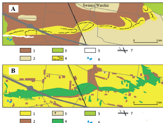
Ryc. 12. Budowa geologiczna i użytkowanie ziemi w okolicach Świnic Warckich A – budowa geologiczna: 1 – glina zwałowa, 2 – eluwia piaszczysto-mułkowe na glinach zwałowych, 3 – piaski teras nadzalewowych, 4 – piaski eoliczne i wydmy z liniami grzbietowymi, 5 – namuły den dolinnych, 6 – zbiorniki wodne, 7 – wybrane drogi i linia kolejowa B – użytkowanie ziemi: 1 – grunty orne, 2 – zabudowa, 3 – cmentarz, 4 – lasy, 5 – łąki, 6 – zbiorniki wodne, 7 – wybrane drogi i linia kolejowa
